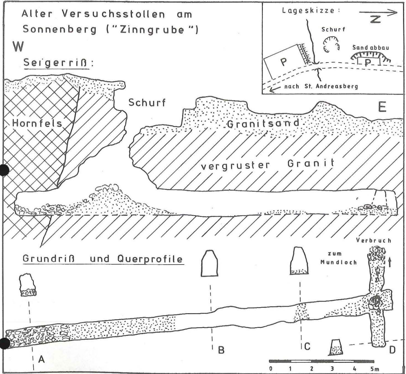
Abb.2 Grund - und Seigerriß des alten Stollens am Sonnenberg
