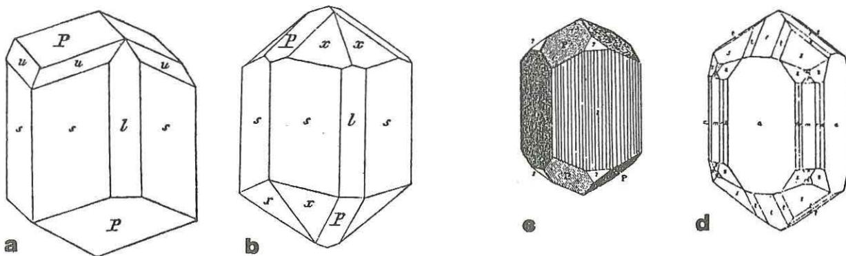
Abb.1 Turmalinkristalle vom Sonnenberg (a,b) und Zinnsteinkristalle aus dem Erzgebirge (c,d). Beide Mineralarten können in Form und Aussehen sehr ähnlich sein. (aus GOLDSCHMIDT,1923)
